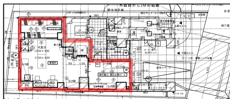
1階平面図
