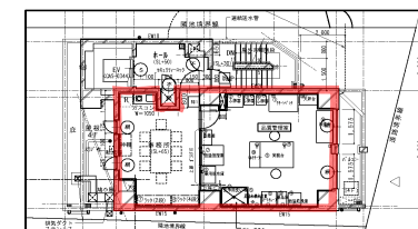
4階平面図
